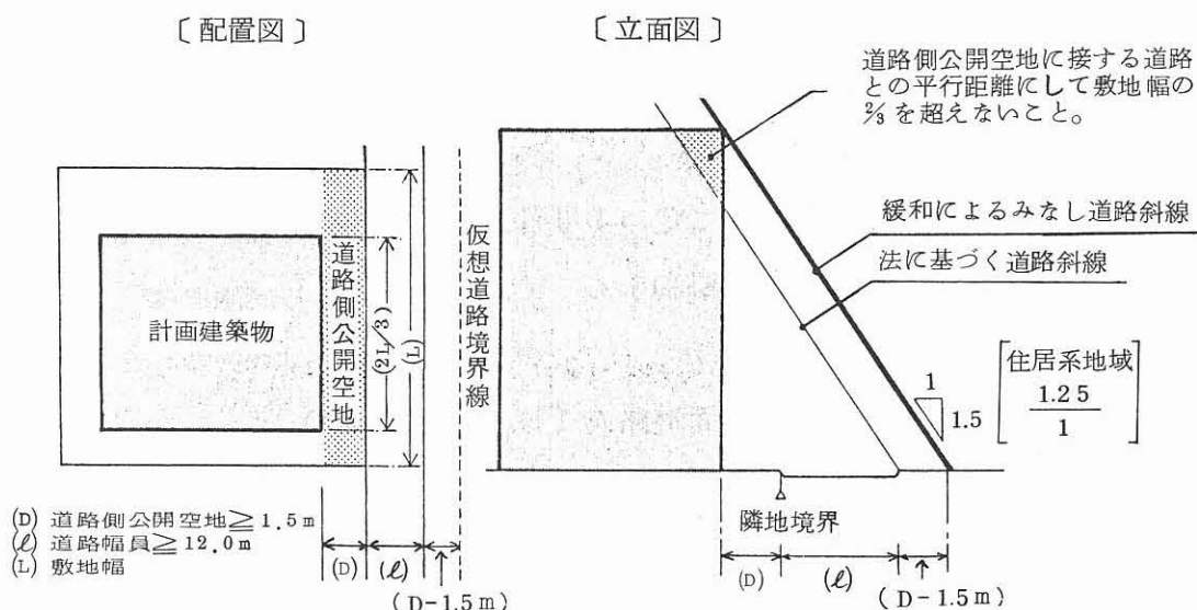
第2図 道路斜線制限の緩和(1) 一方向に道路を有する場合（一般例）
