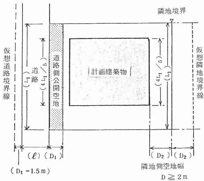
第5-2図 斜線制限緩和の特例
