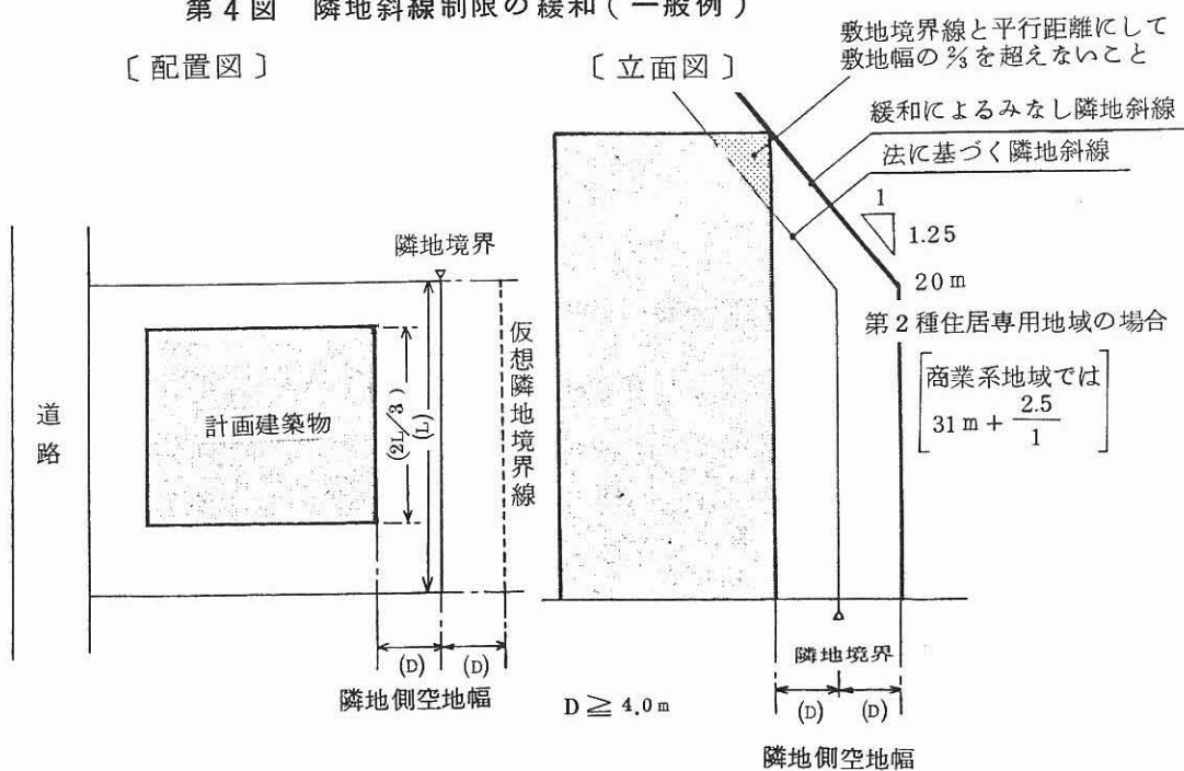
第4図 隣地斜線制限の緩和(一般例)
