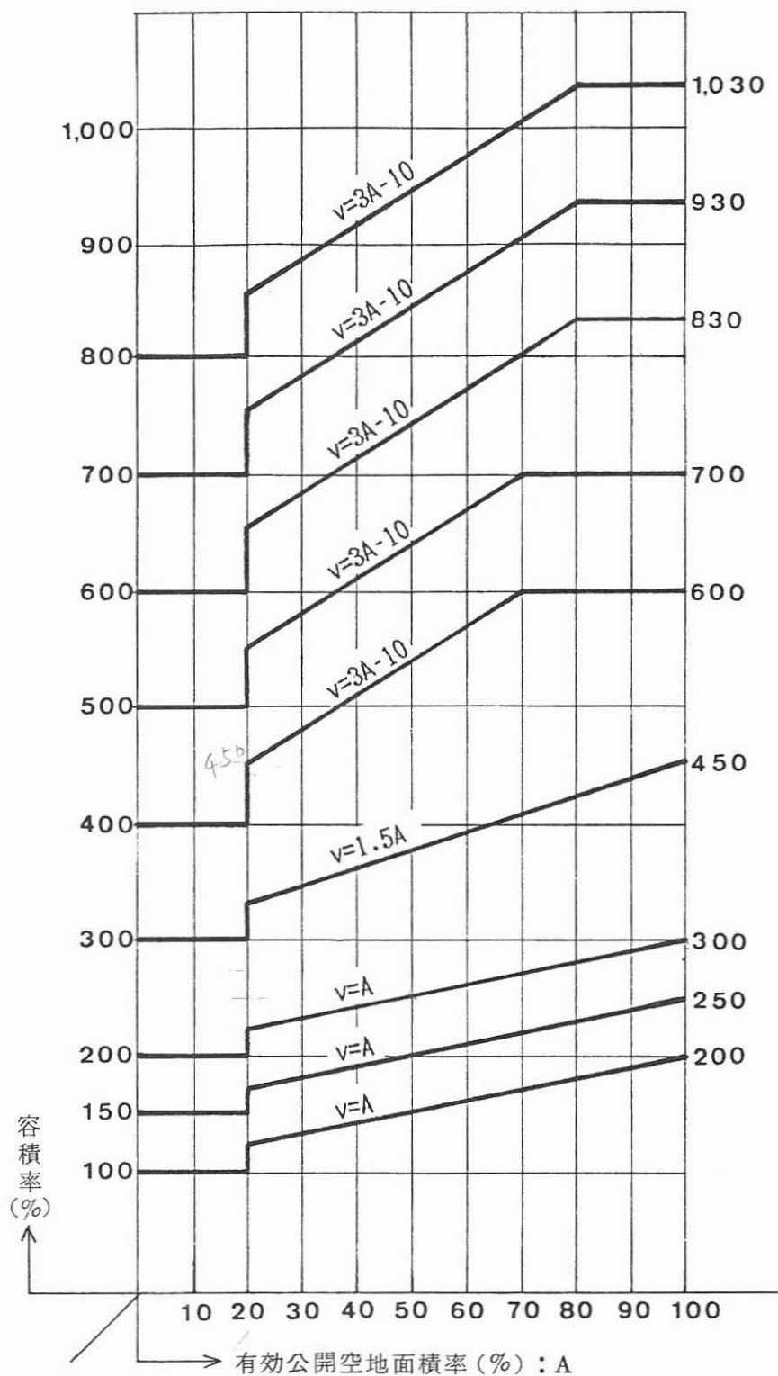
第1図 容積率割増のグラフ
