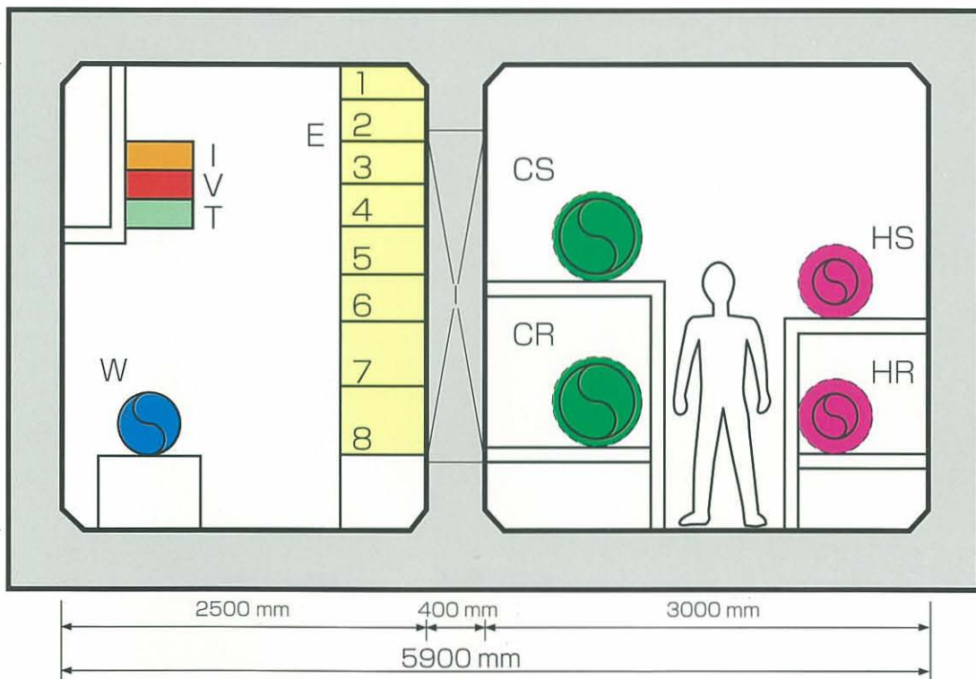
複断面タイプ (収容対象物件を全て収容するタイプ)
