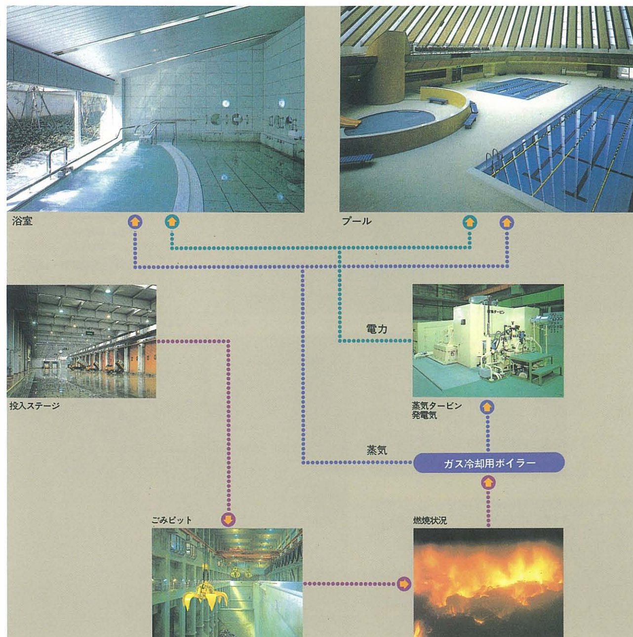
北部工場と 余熱利用のしくみ
